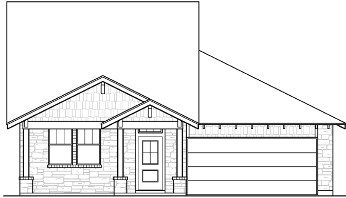
ELEVATION A
