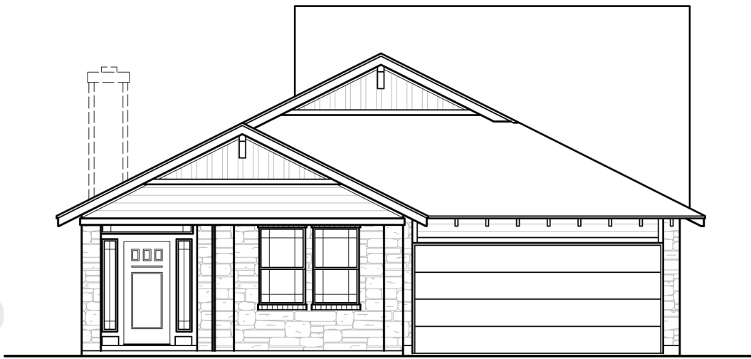
ELEVATION B
